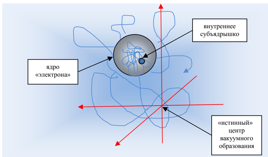
Рис. 2.9.1. Хаотически блуждающее ядро «электрона», внутри которого хаотически блуждает внутренне субъядрышко
