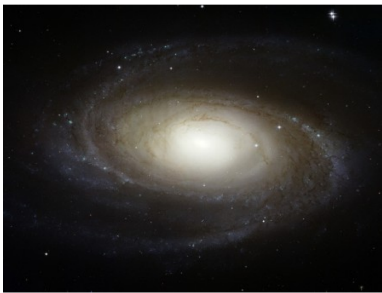
Спиральная галактика M81 (Hubble) (фото: www.img1.gelz.net )
