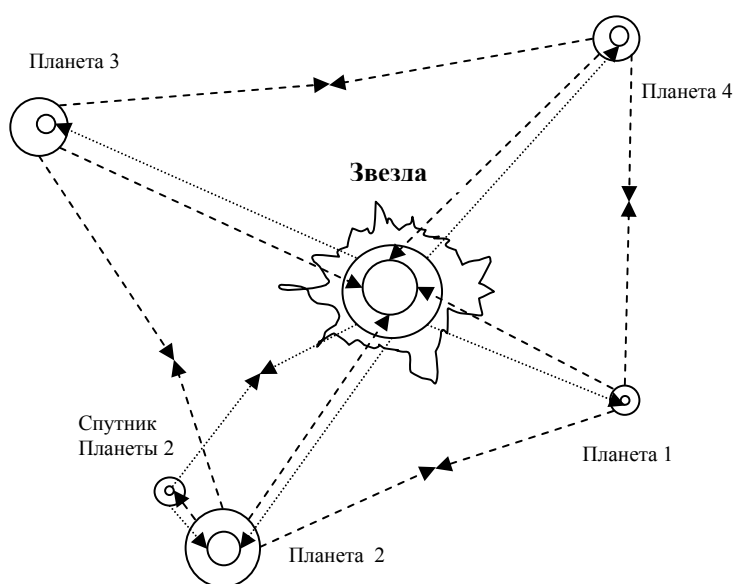
Рис. 3.3.1. «Звездно-планетарная» система, где .....> – усредненные направления течений субконта ; ---> – усредненные направления течений антисубконта
