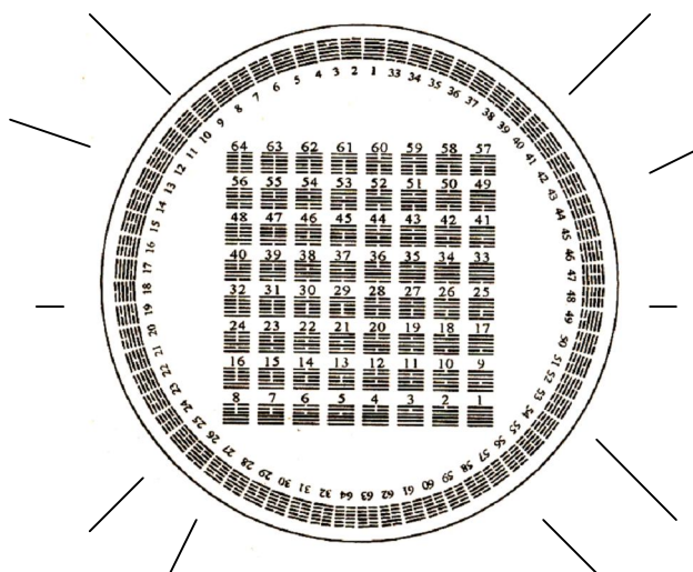
Рис. 28. Эволюция Тай-Цзи (Великого Предела)
